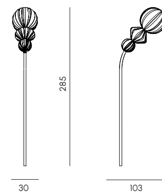
Joy lampione senza base Joy pathway lamp post without base
